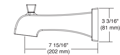
RP77091▲ (Pull-Up Diverter)
