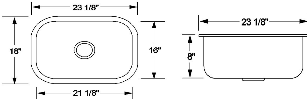
Sink Strainer Optional
