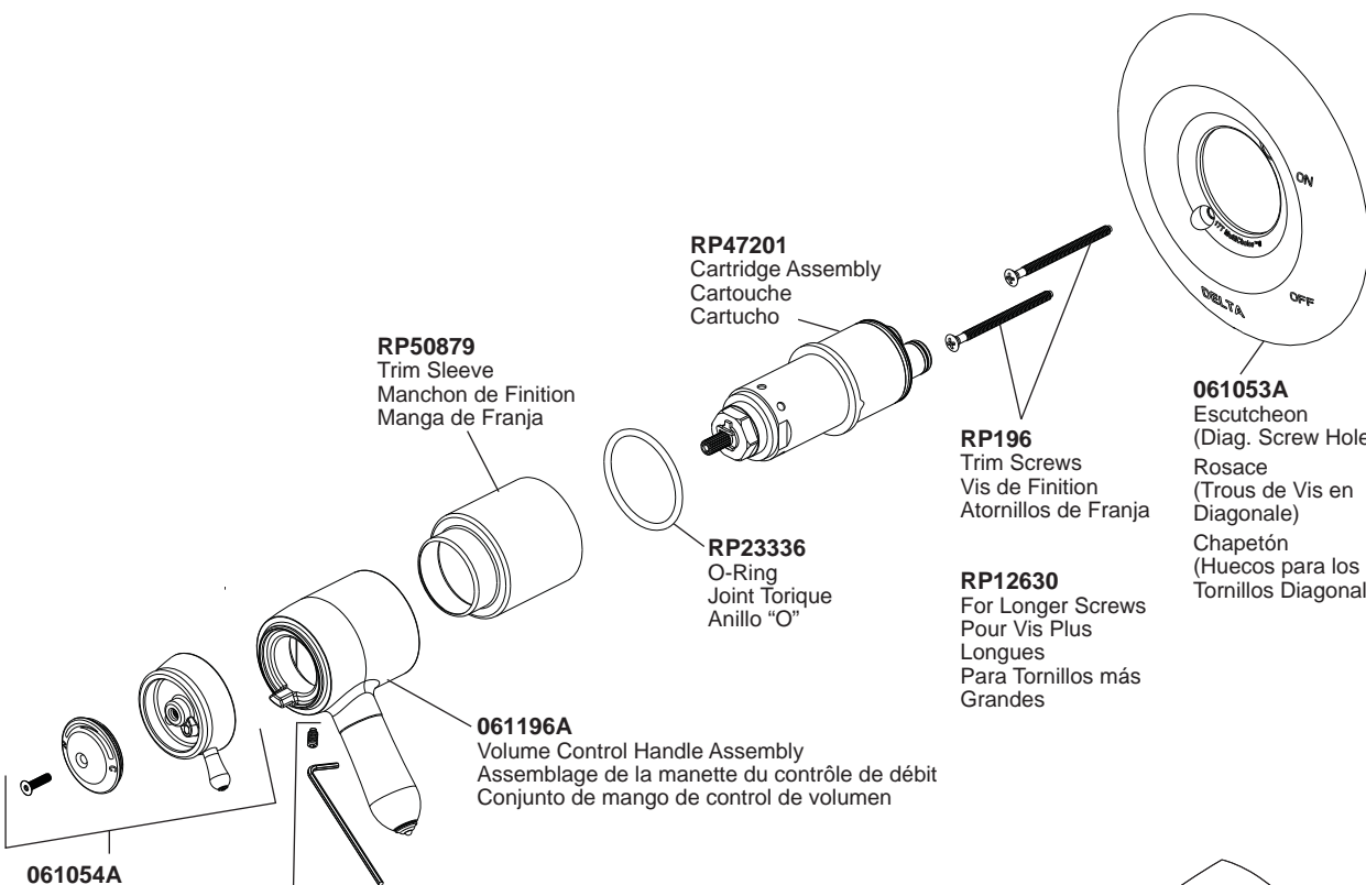
RP50465 Set Screw & Wrench Vis de Calage et Clé Tornillo de Ajuste y Llave
