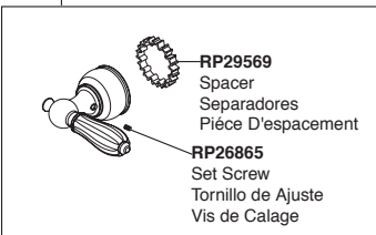
H712 ▲ Handle Kit Juego de herrajes de la Manija Manette en kit
