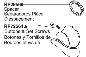
H798▲ Handle Kit Juego de herrajes de la Manija Manette en kit
