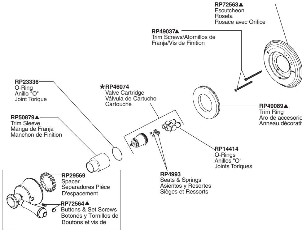
H797▲ Handle Kit Juego de herrajes de la Manija Manette en kit
