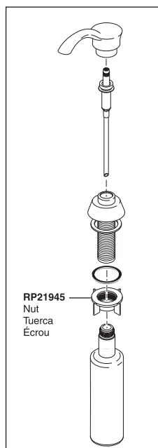
RP50781▲ Dispenser Assembly Ensamble del Dispensador Distributeur
