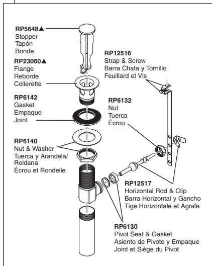
RP26533▲ Metal Pop-Up Assembly Ensamble de Metal del Desagüe Automático Renvoi Mécanique en Métal
