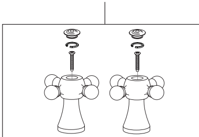
RP52400▲ Cross Handle w/Button, Friction Ring & Set Screw Manija con Botón, Arandela de Fricción y Tornillo de Ajuste Manette avec Bouton, Rondelle de Friction et Vis de Calage
