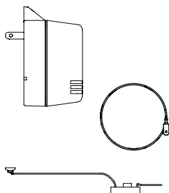
La opción de transformador conectable (PT) incluye un transformador (S53-338), adaptador (S53-339) y kit de conexión a tierra (S53-349) para las llaves CAP-DCR
