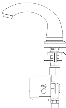
Llave capacitiva serie 1200* (S53-315)
